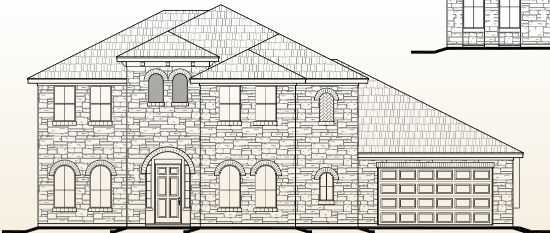
Elevation B
